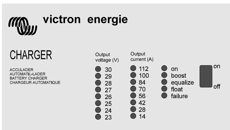
Obrázek 5. Příklad předního panelu nabíječky baterií.
