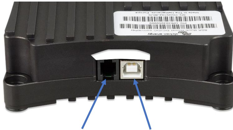
CAN.Bus aansluiting (niet voor het 25 A-model)
